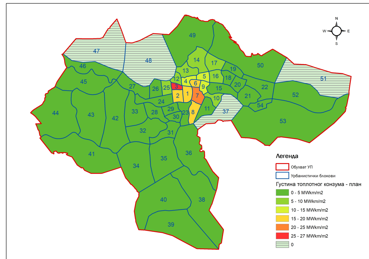
Слика 1. Просторна расподела густине топлотног конзума
