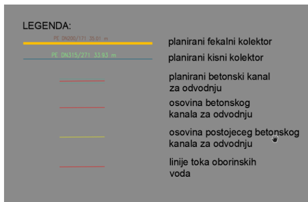
Slika 8. Pregledna situacija kanalizacionog sistema upotrebljenih i atmosferskih voda u naselju Police (Gornje Police)
